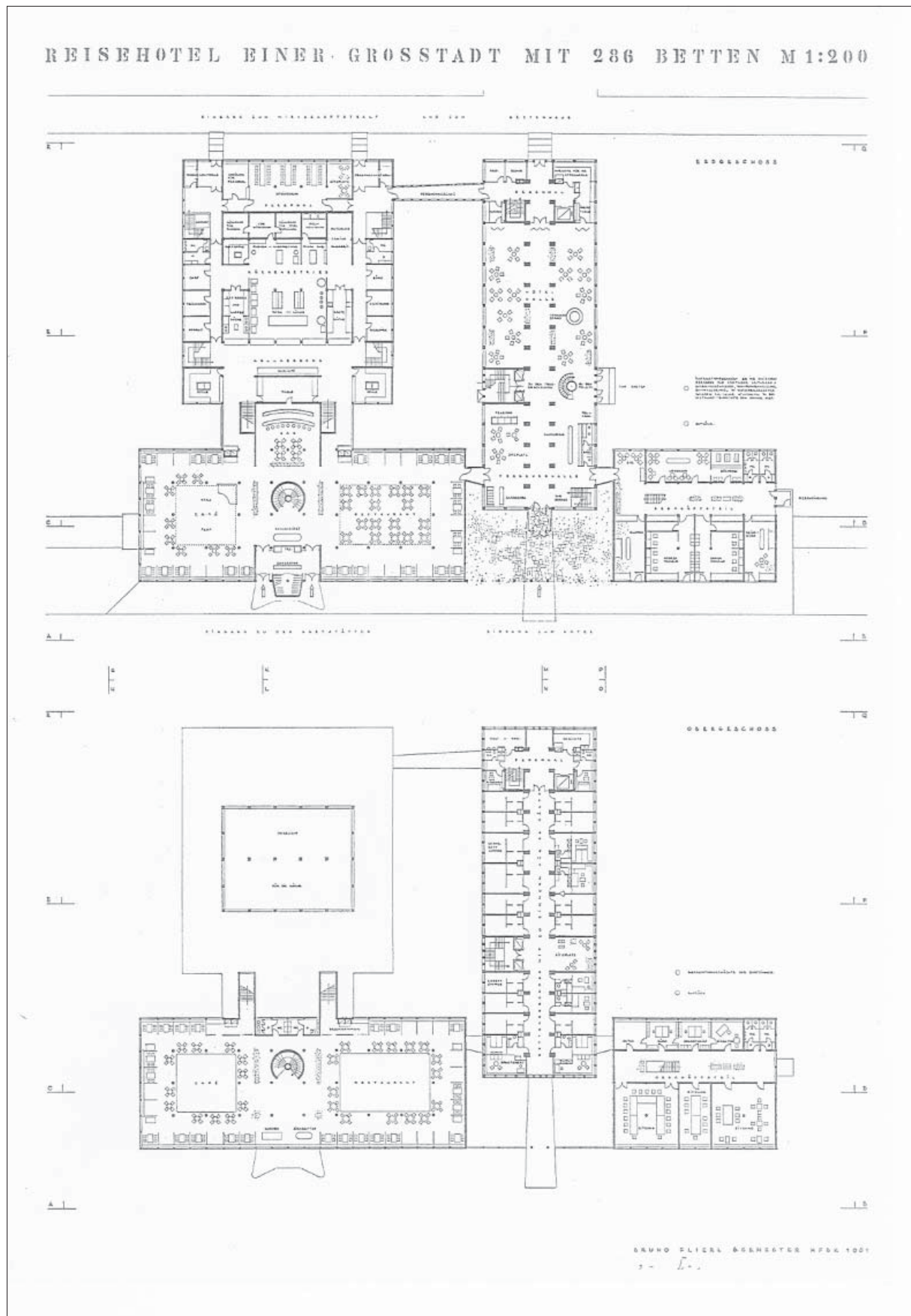
Abb. 3: Studentenentwurf HfBK 1951. Reisehotel. Grundrisse Erdgeschoss und Obergeschoss
