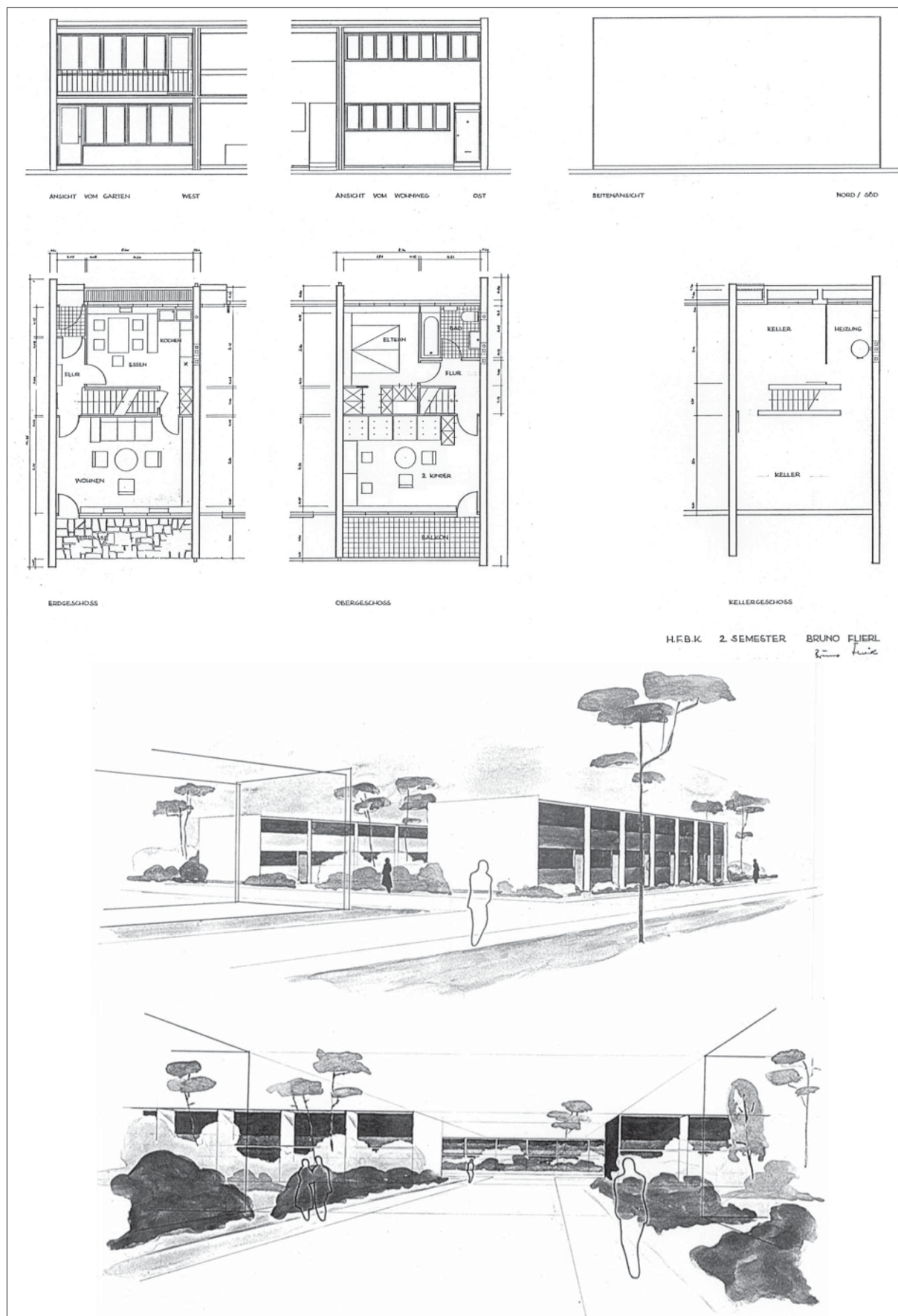
Abb. 1: Studentenentwurf HfBK 1949. Zweistöckiges Einfamilien-Reihenhaus 4 Betten, Typ Quertreppe. Ansichten, Grundrisse Erdgeschoss, Obergeschoss und Kellergeschoss, Perspektiven
