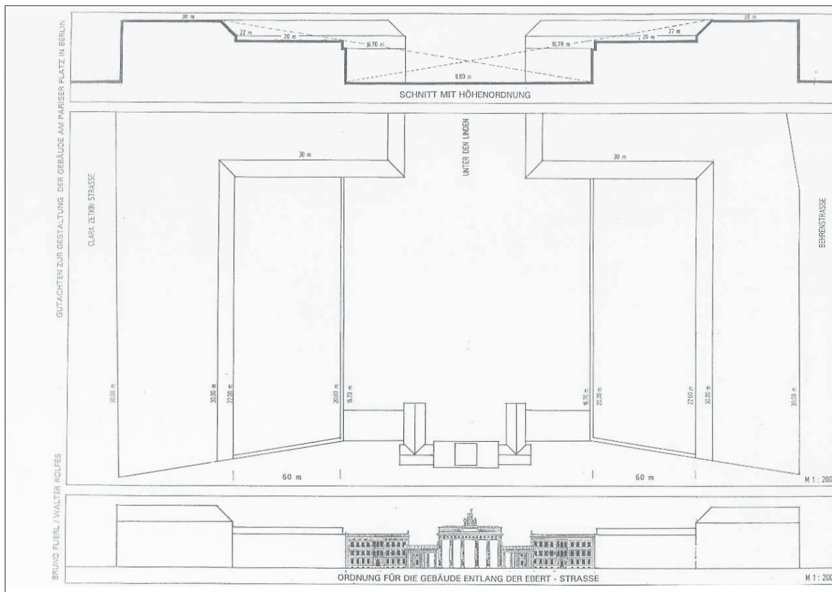
Abb. 32: Gutachten Pariser Platz: Schnitte mit Höhenordnung
